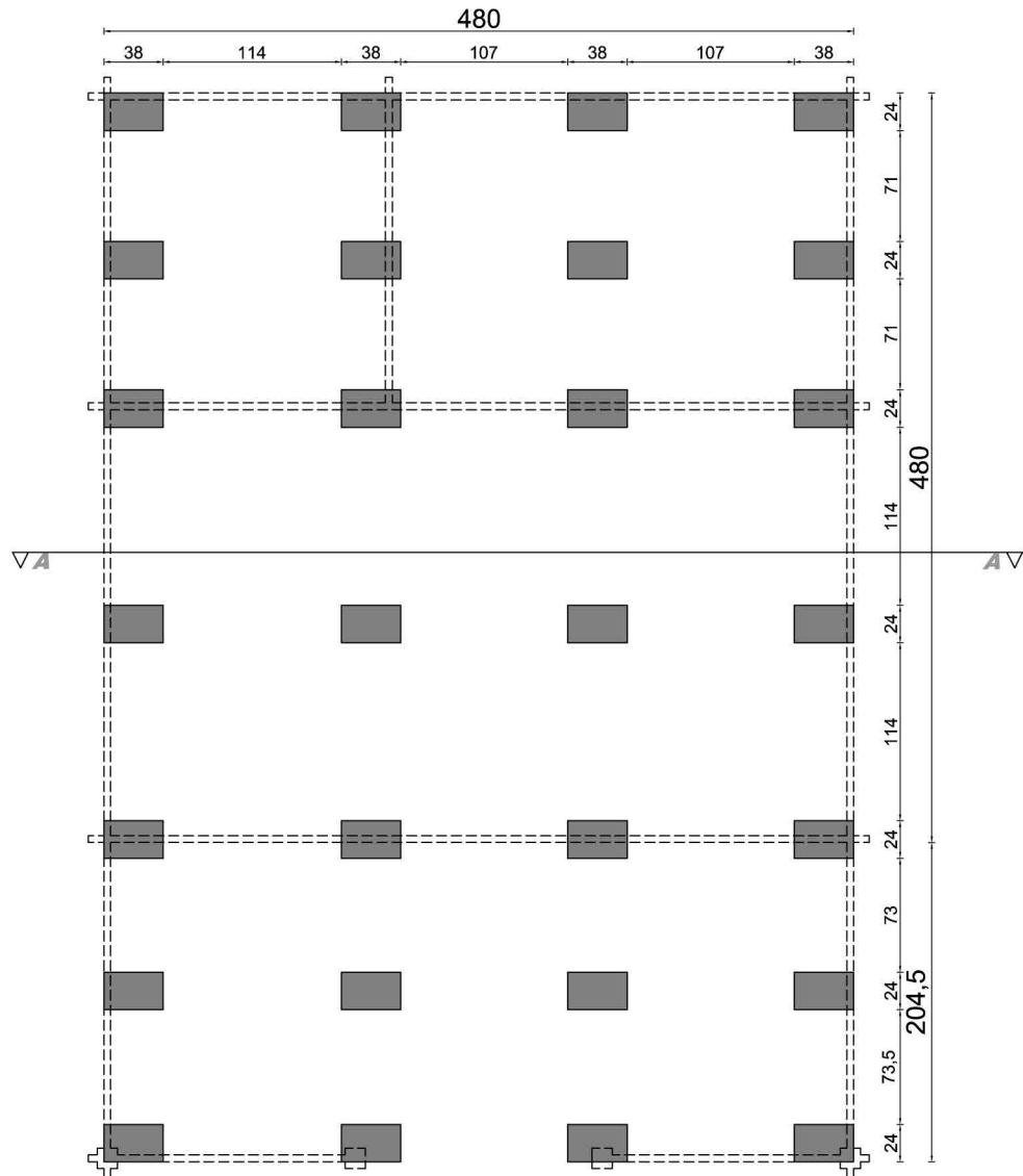
rzut fundamentów
