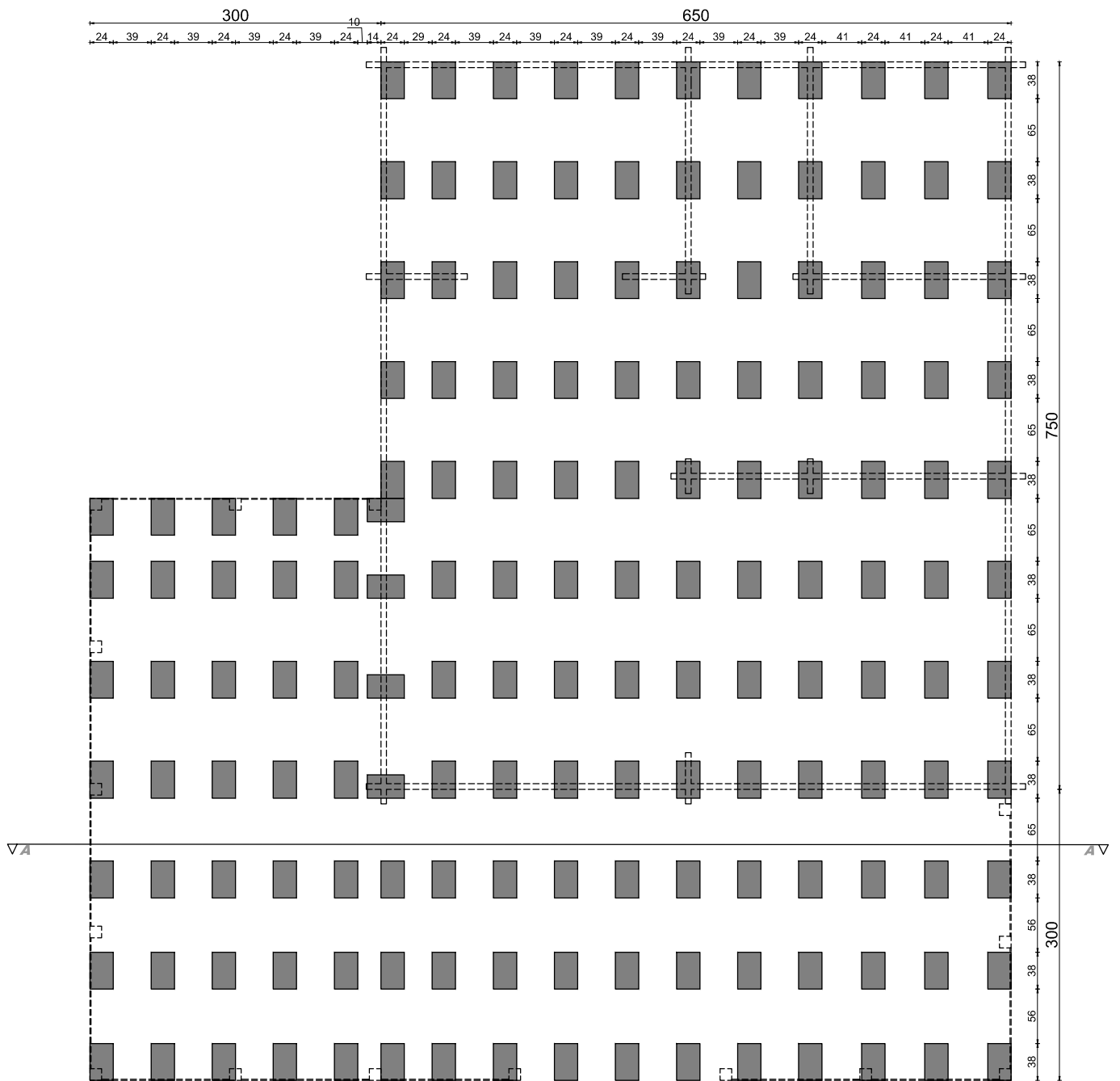
rzut fundamentów
