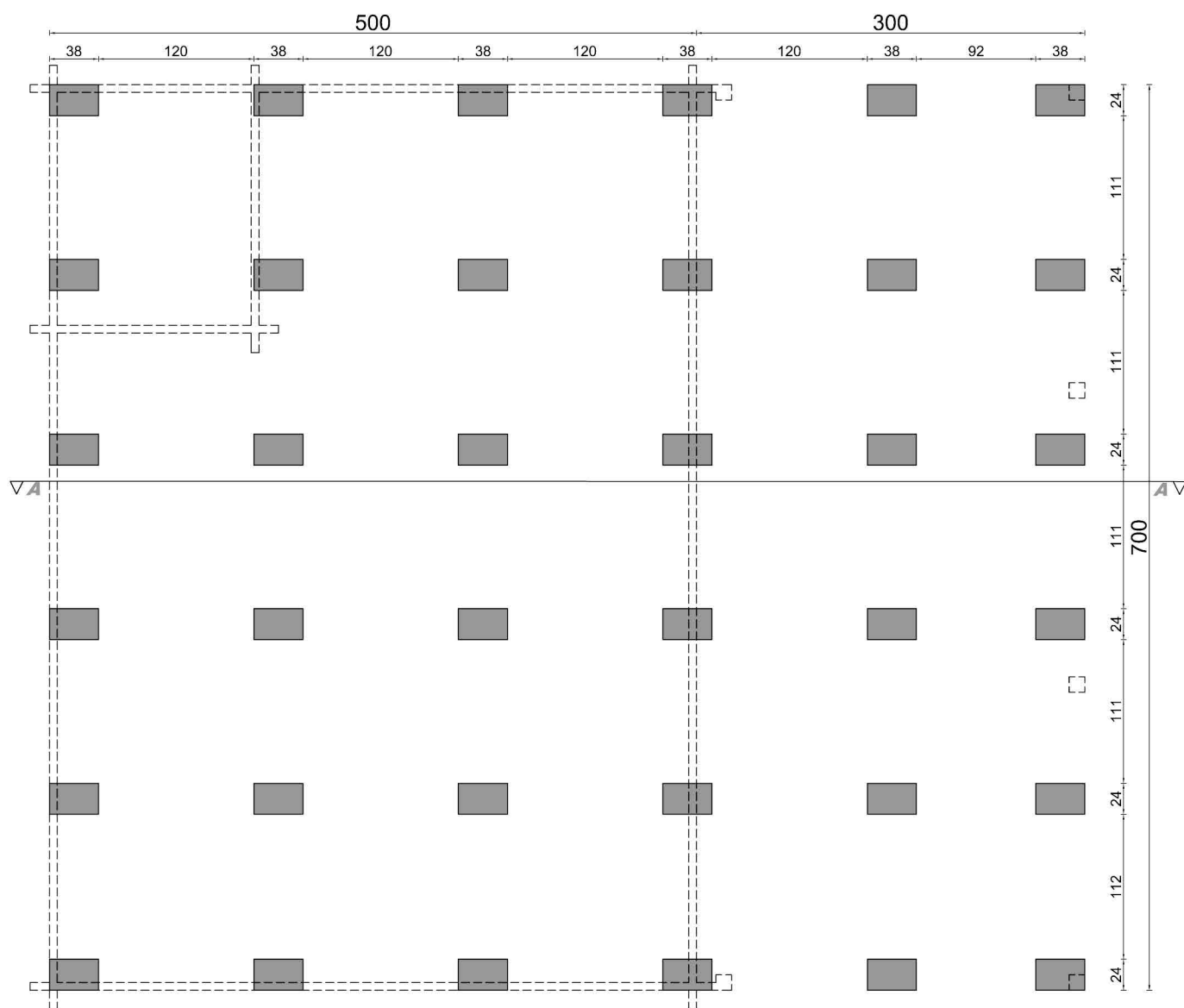
rzut fundamentów
