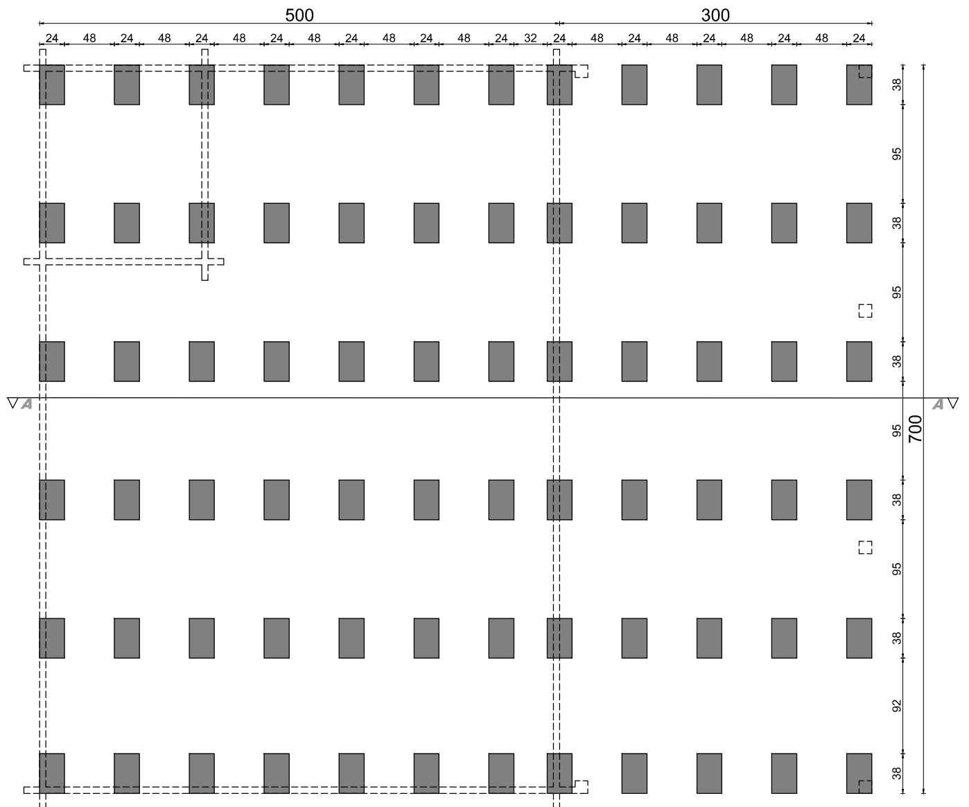
rzut fundamentów
