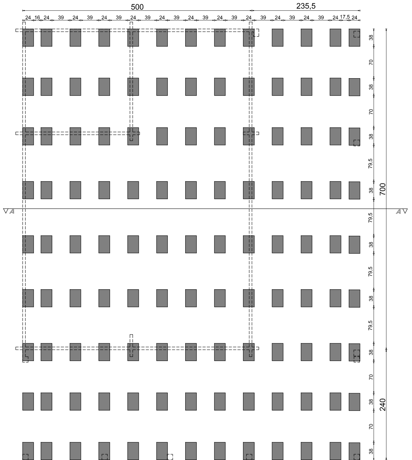
rzut fundamentów
